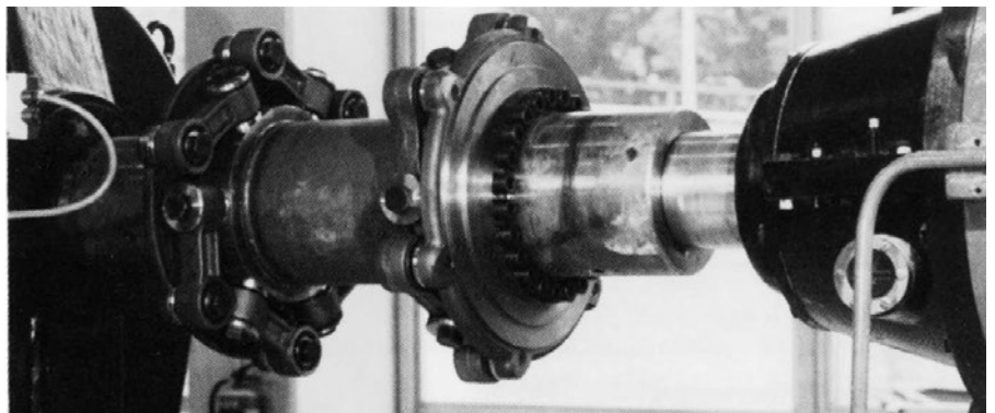
CENTALINK-Gelenkwelle in 500 kW Windkraftwerk.
